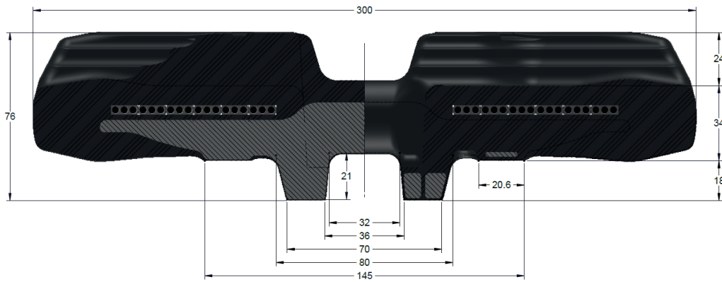
QUERSCHNITT
