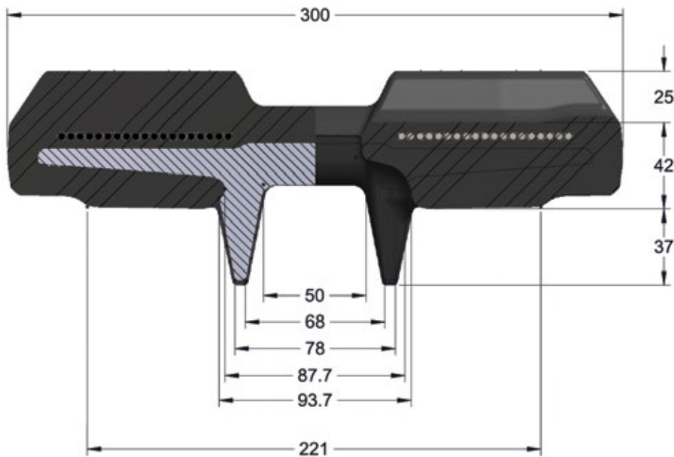
QUERSCHNITT
